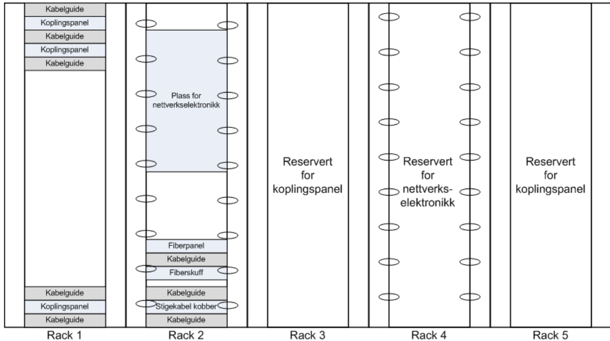
Figur 2 Rackrad i kommunikasjonsrom
